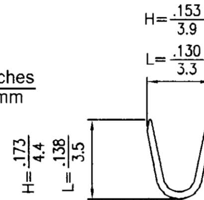
A-A SECTION
