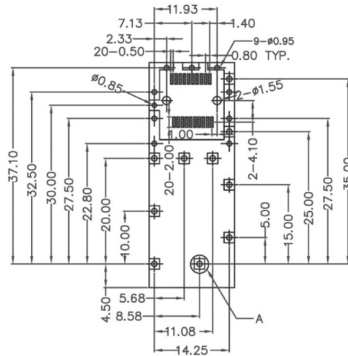
P.C.B LAYOUT TOP VIEW \pm 0.05
