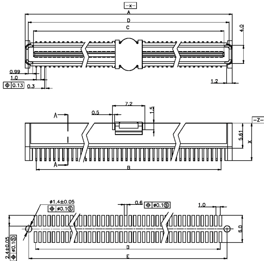
P.C.Board Layout
