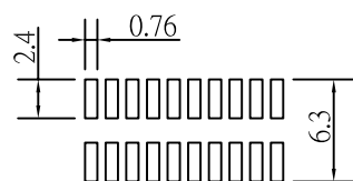
P.C.Board Layout
