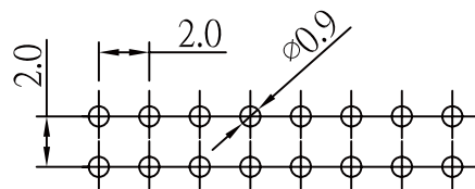
P.C.Board Layout
