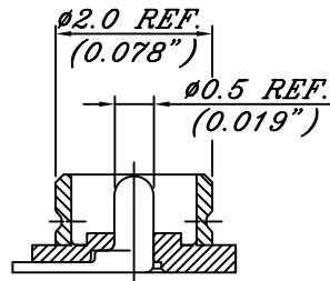
A-A SECTION
