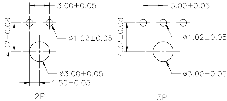
P.C.B LAYOUT
