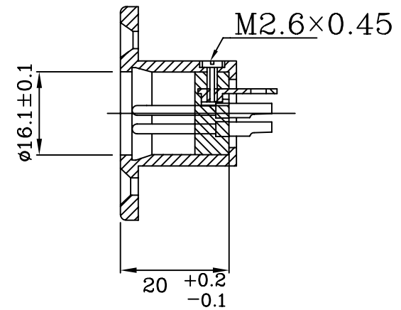
A-A SECTION
