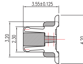
D-D
