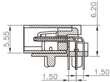
SEC: A-A
