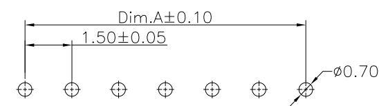
P.C.B Layout
