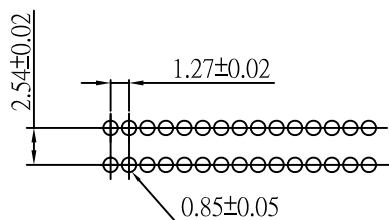
P.C.Board Layout
