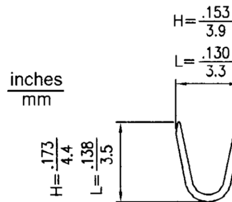
A-A SECTION
