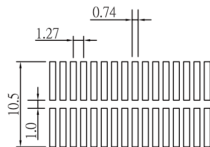
P.C.Board Layout
