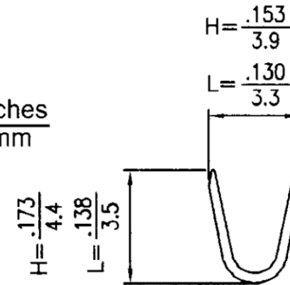
A-A SECTION
