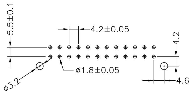
P.C.B. LAYOUT
