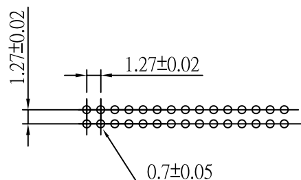
P.C.Board Layout
