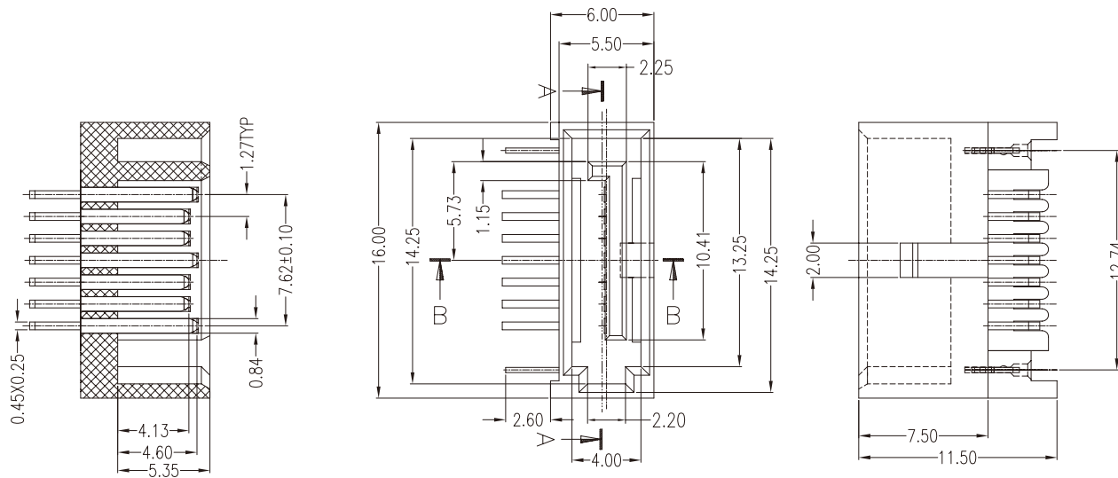
SECT A-A
