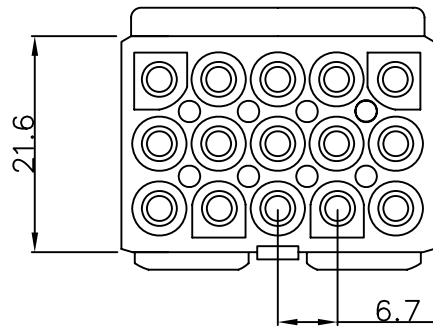
PWL-P-3X05
