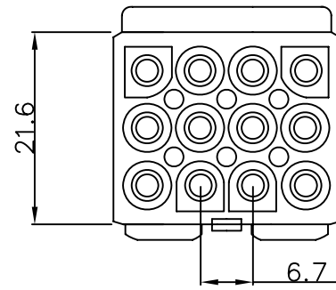
PWL-P-3X04
