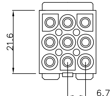
PWL-P-3X03
