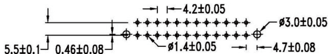
P.C.B. hole dimensions
