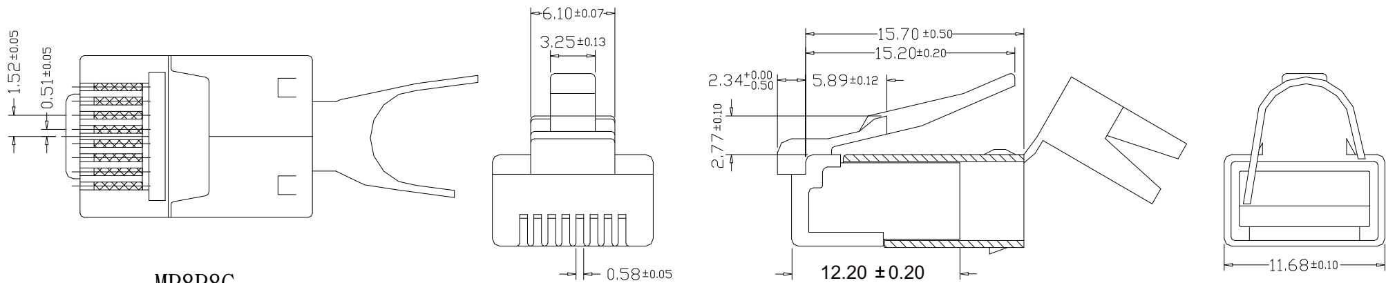
MP8P8C
