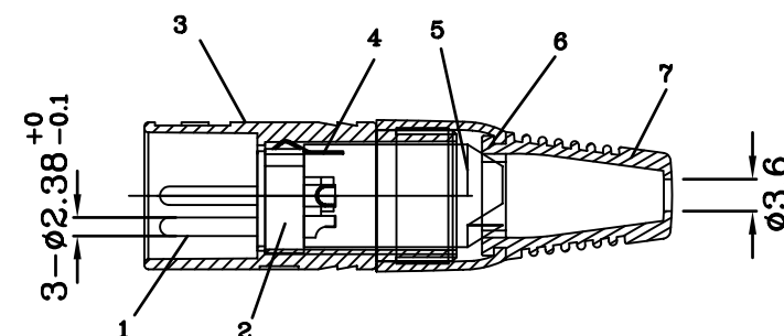
A-A SECTION
