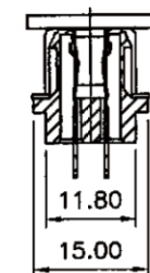
A-A SECTION
