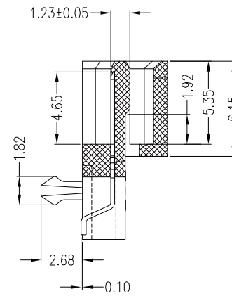
SECT A-A
