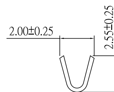
A-A SECTION
