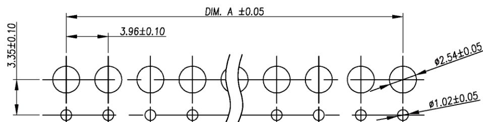
P.C.B LAYOUT
