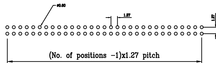
P.C.B. layout
