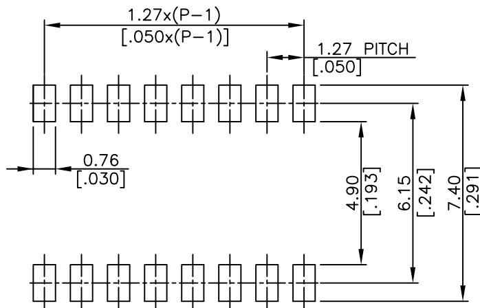
P.C.B LAYOUT
