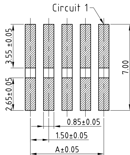
P.C.B LAYOUT
