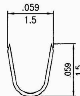
A-A SECTION
