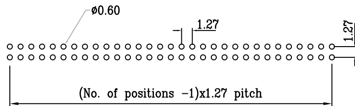
P.C.B. layout
