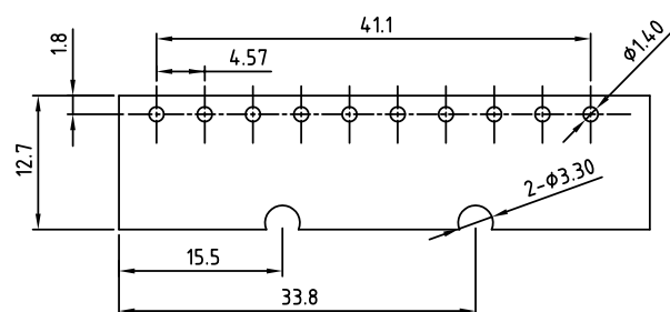
P.C.B Layout
