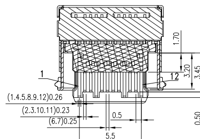
SECTION B-B(SC 1:1)
