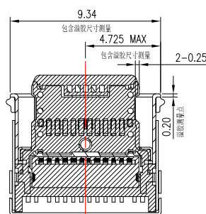
SECTION A-A(SC 1:1)
