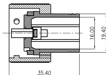
防水HDMI(M) 成品(BLACK)A TYPE
