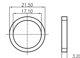
扁型 O-RING(17.1*2.2*3.2
