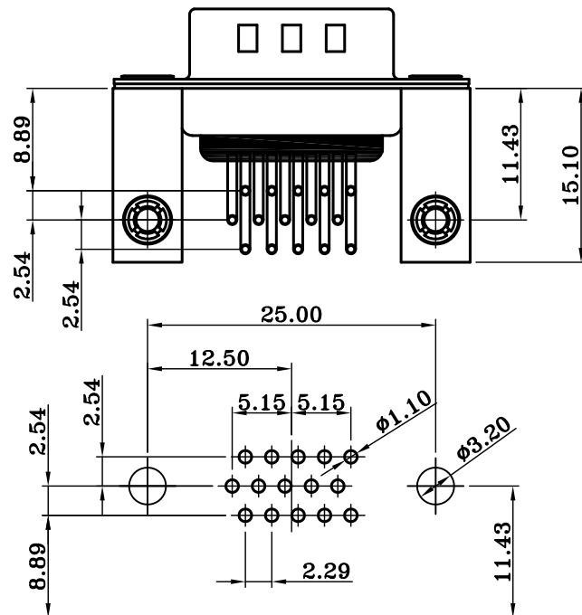
P.C.B LAYOUT
