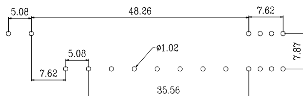
P.C.B. layout
