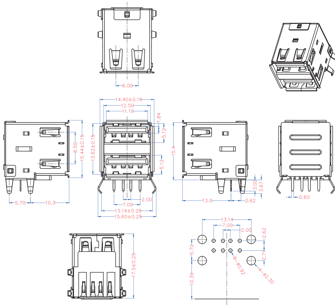
RECOMMEND P.C.B. LAYOUT
