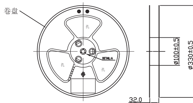
卷帶盤(圖一)
