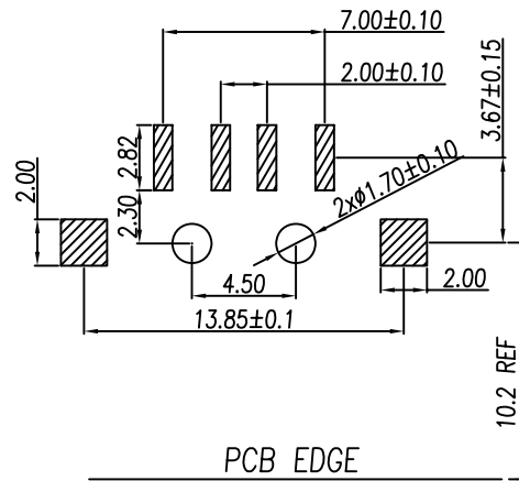
P.C.B. PATTERN LAYOUT
