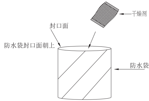
④ 10盘产品入防水袋示意图
