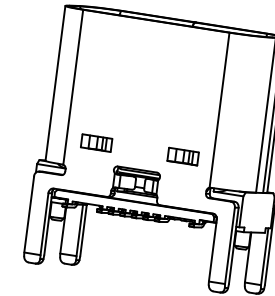
外壳脚长度规格: DIM A
