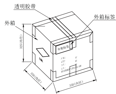
外箱尺寸为内径, 单位:mm
