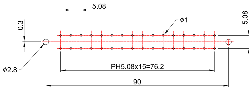
P.C.B LAYOUT
