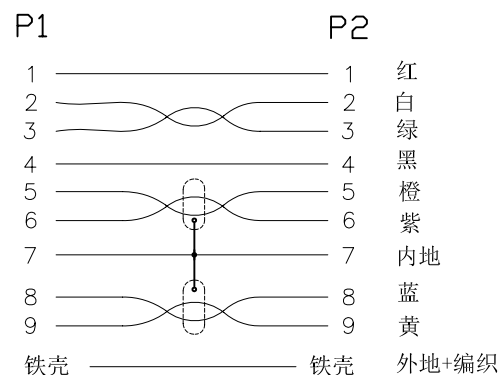
接线图
