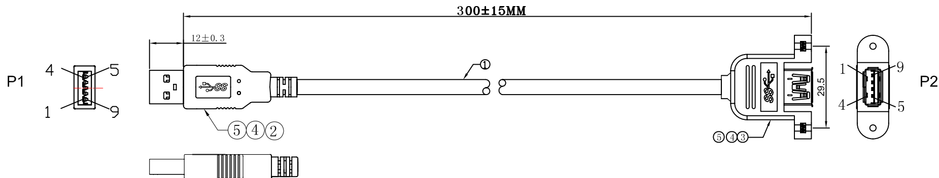
接线图
