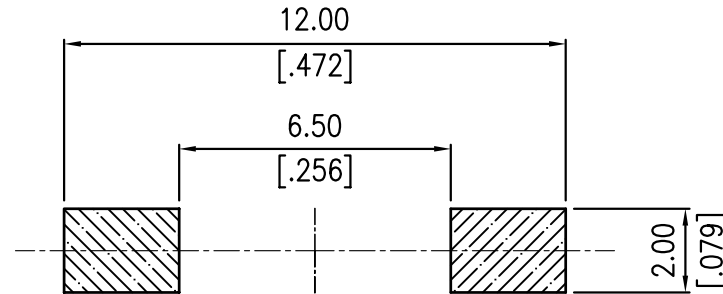
P.C.B. LAYOUT
