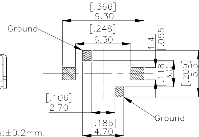
P.C.B. LAYOUT
