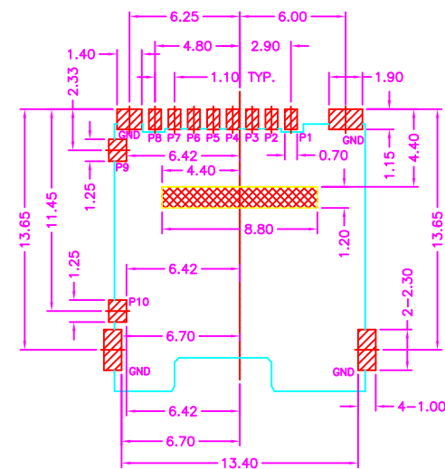
P.C.B LAYOUT TOP VIEW \pm 0.05
