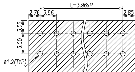
P.C.B. LAYOUT(REF)
