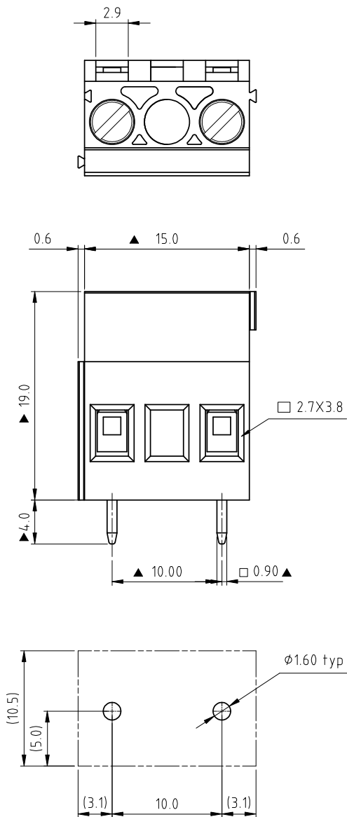
P.C.B. LAYOUT
